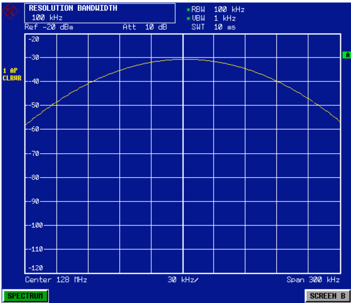
Bild 5-5 Messung von zwei gleich großen HF-Sinussignalen mit einer Auflösebandbreite, die größer als deren Frequenzabstand ist.
