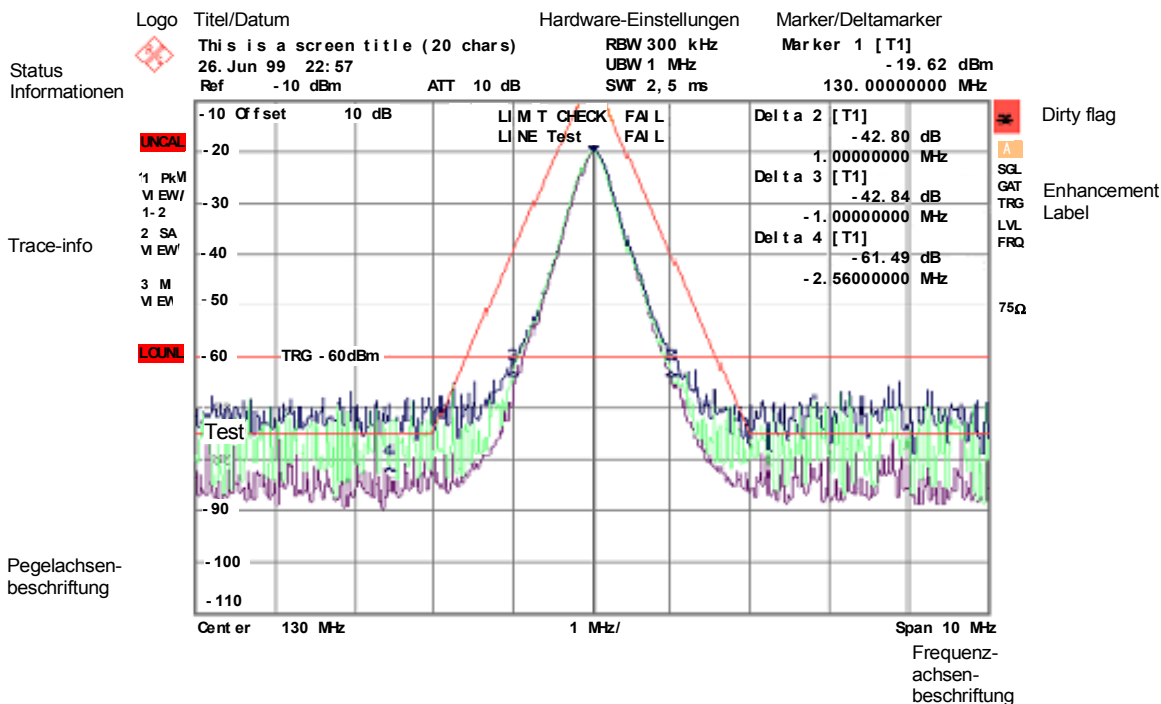
Bild 4-1 Bildschirmaufteilung des R&S FSP im Analysatorbetrieb
