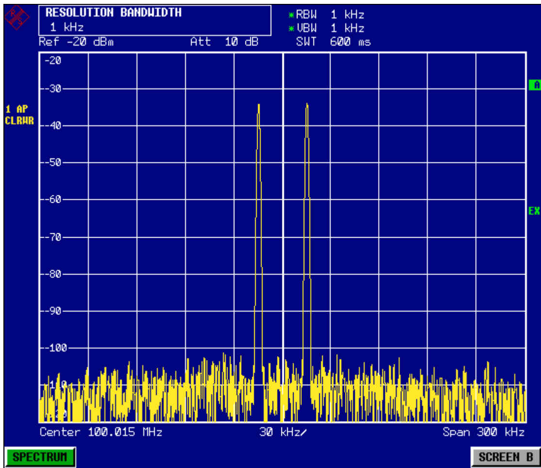
Bild 5-6 Messung von zwei gleich großen HF-Sinussignalen mit einer Auflösebandbreite (1 kHz), die deutlich kleiner ist als deren Frequenzabstand.
